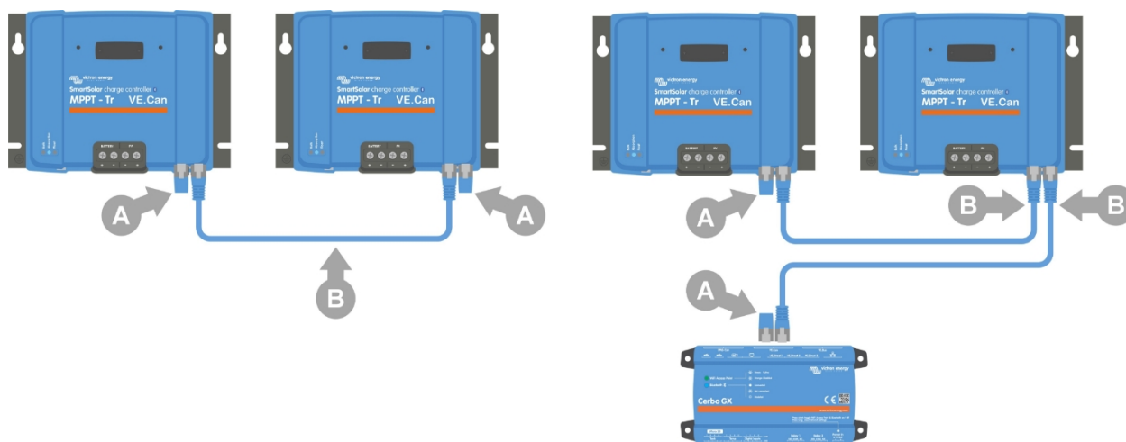
A: terminátor VE.Can - B: kabel RJ45 UTP.
