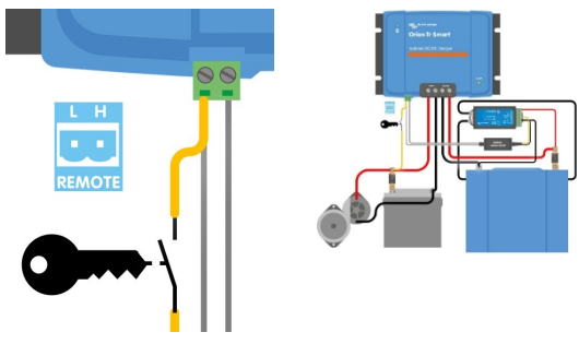
Obrázek 4: Schéma zapojení detekce vypnutí motoru
