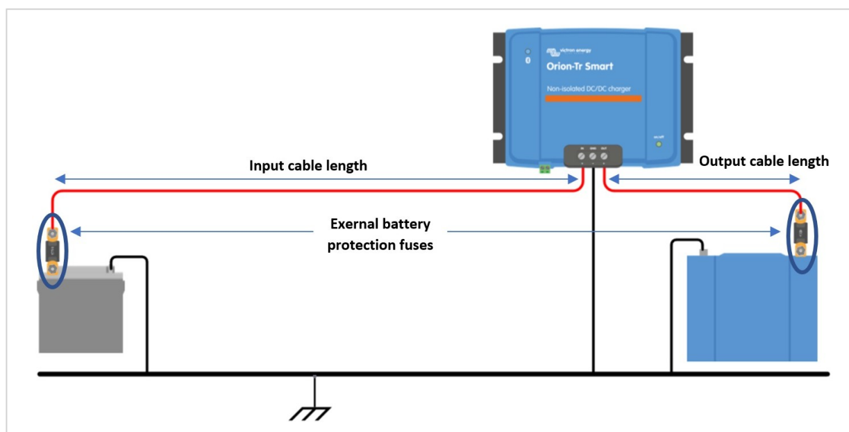
Obrázek 6: Doporučení pro kabely a pojistky
