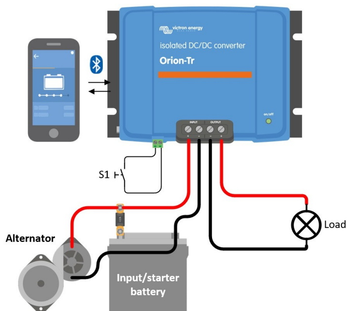
Obrázek 1: Typické zapojení měniče DC-DC
