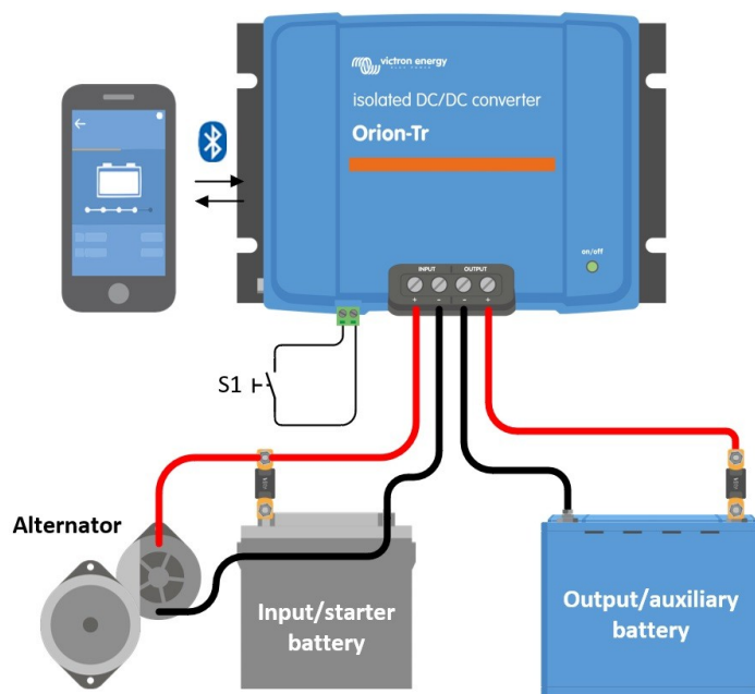
Obrázek 2: Typické nastavení připojení jako nabíječka
