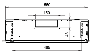
ŘEZ A-A
